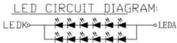
背光电路图
