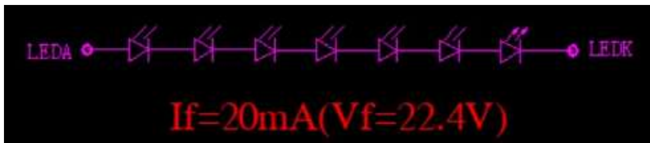
背光电路图
